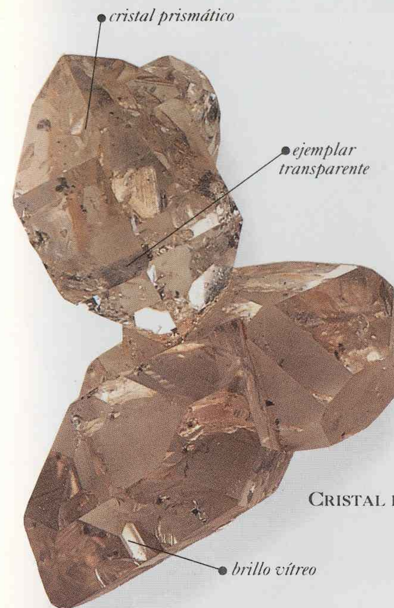
CUARZO LECHOZO
