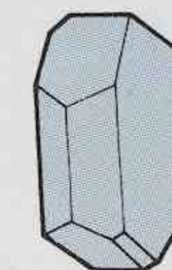
TRICLINICO
