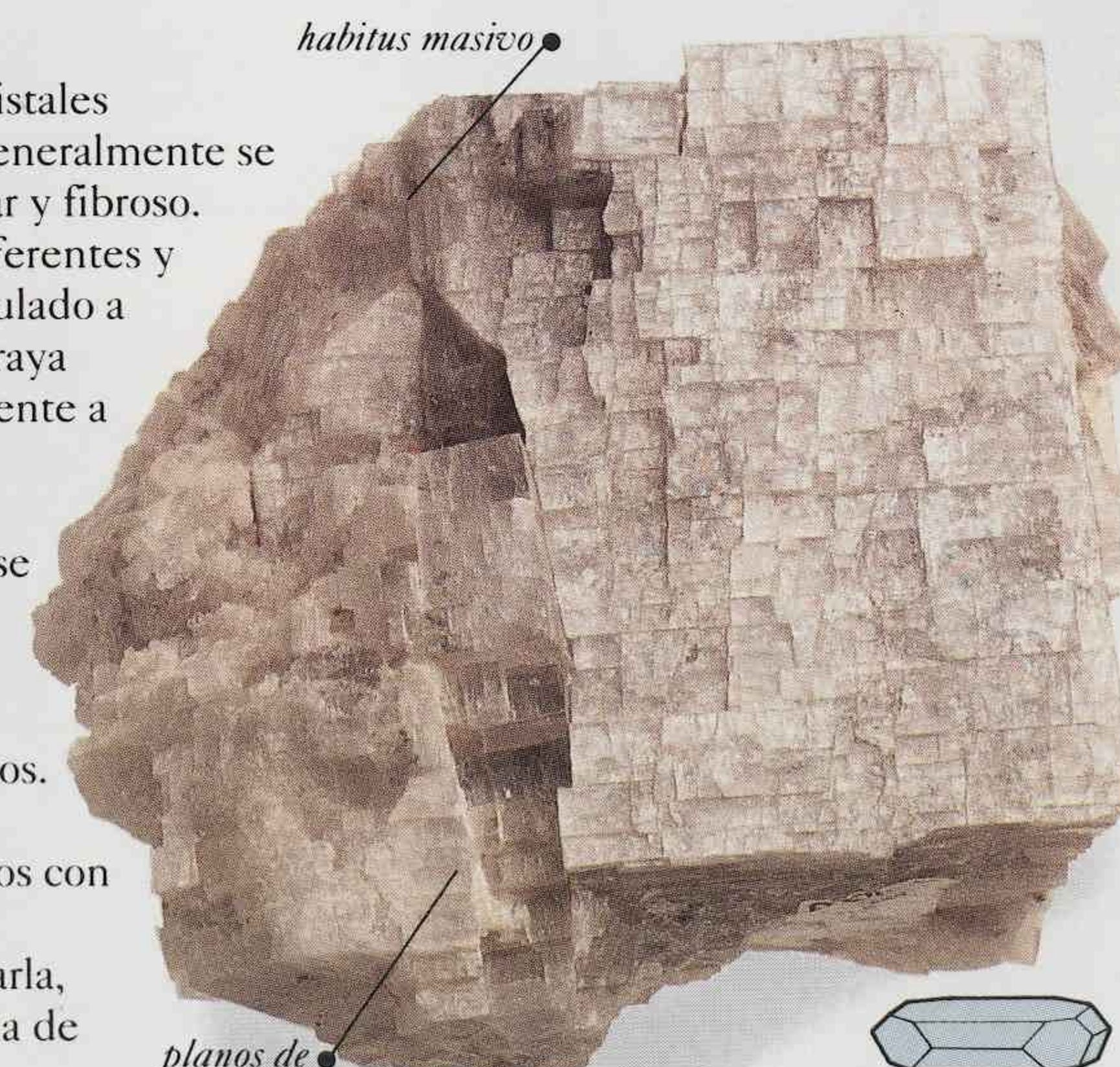
ROMBICO
