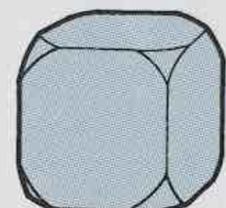
CUBICO
