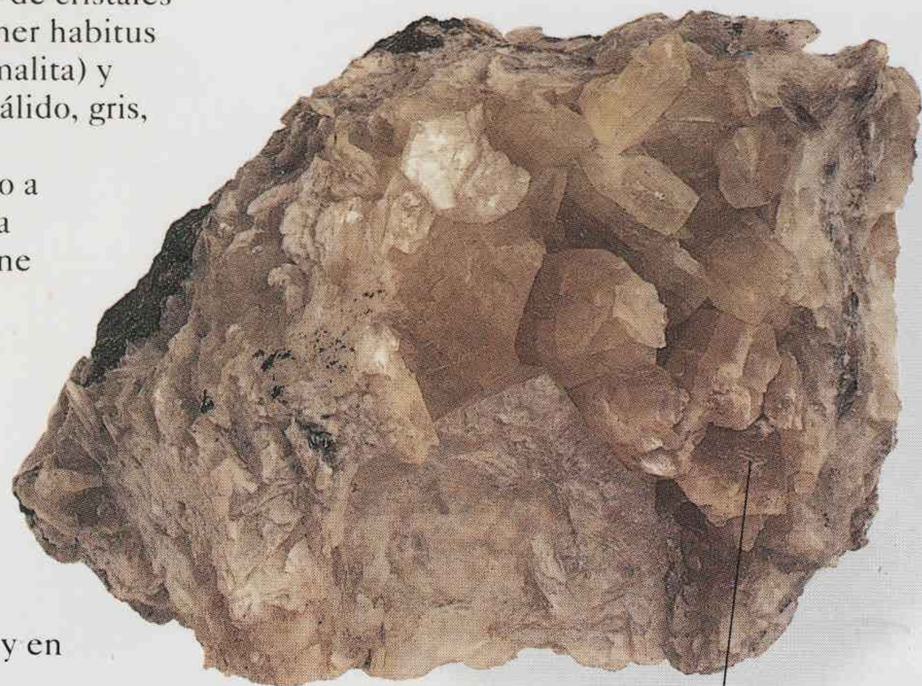
● cristal tabular
