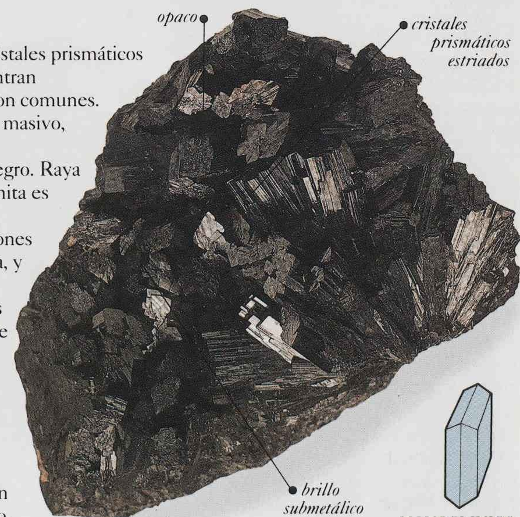
MONOCLINICO
