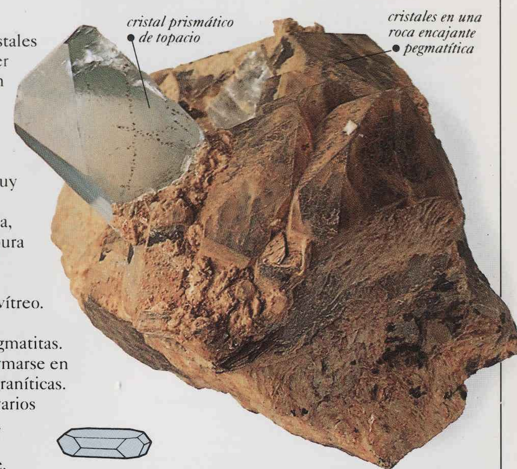
ROMBICO
