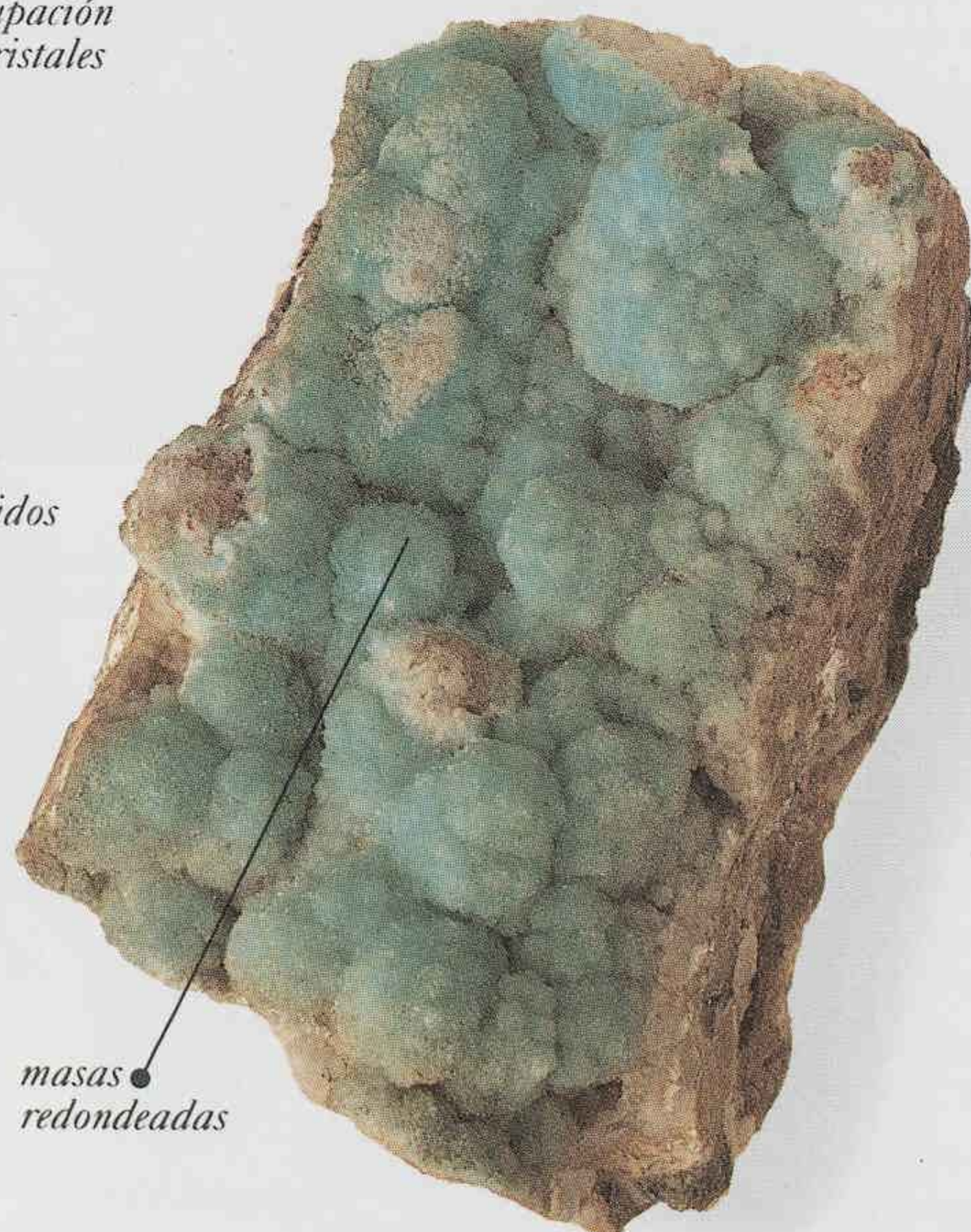
HEMIMORFITA VERDE
