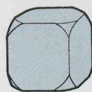
CUBICO
