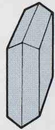
MONOCLINICO
