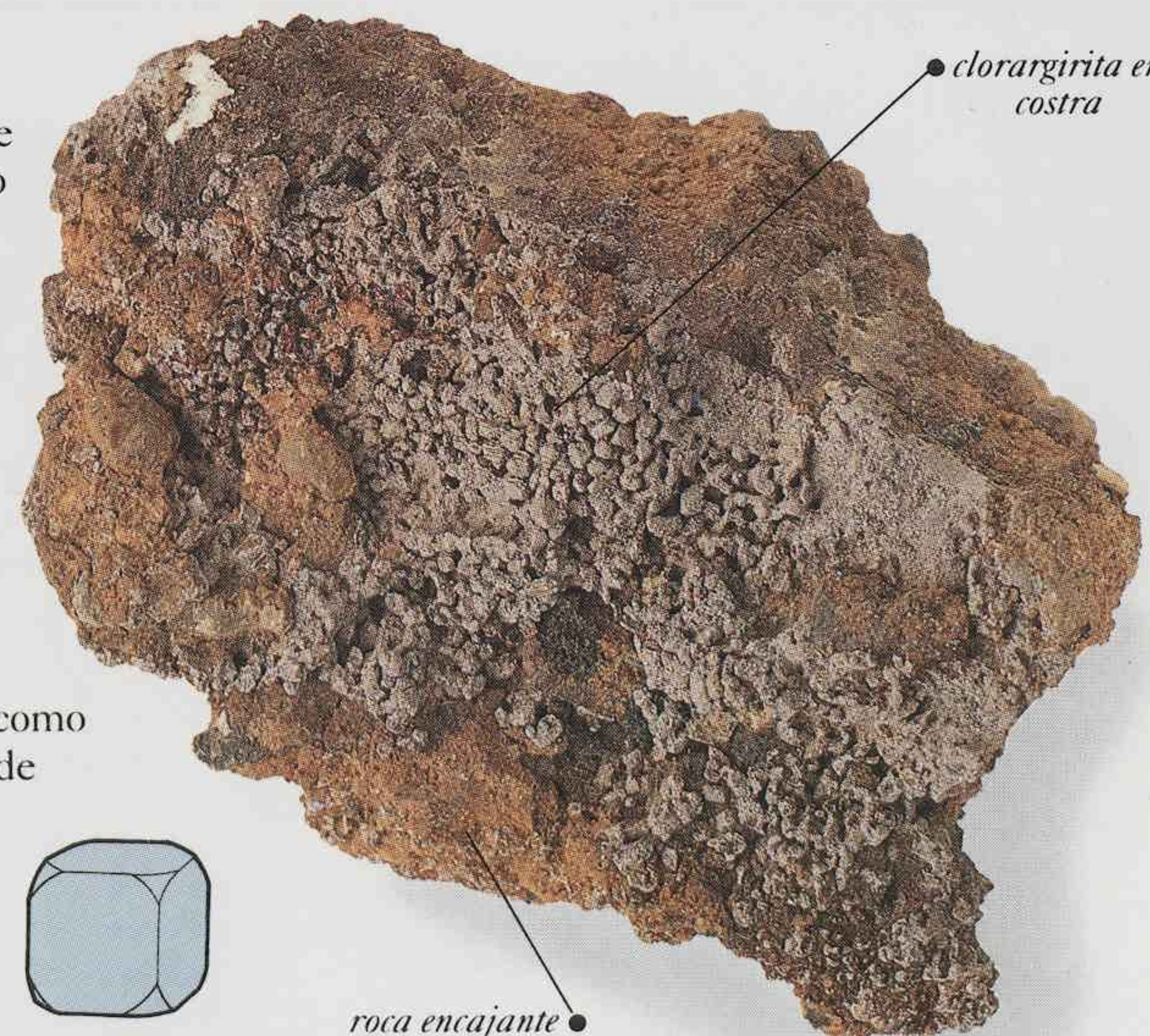
CUBICO
