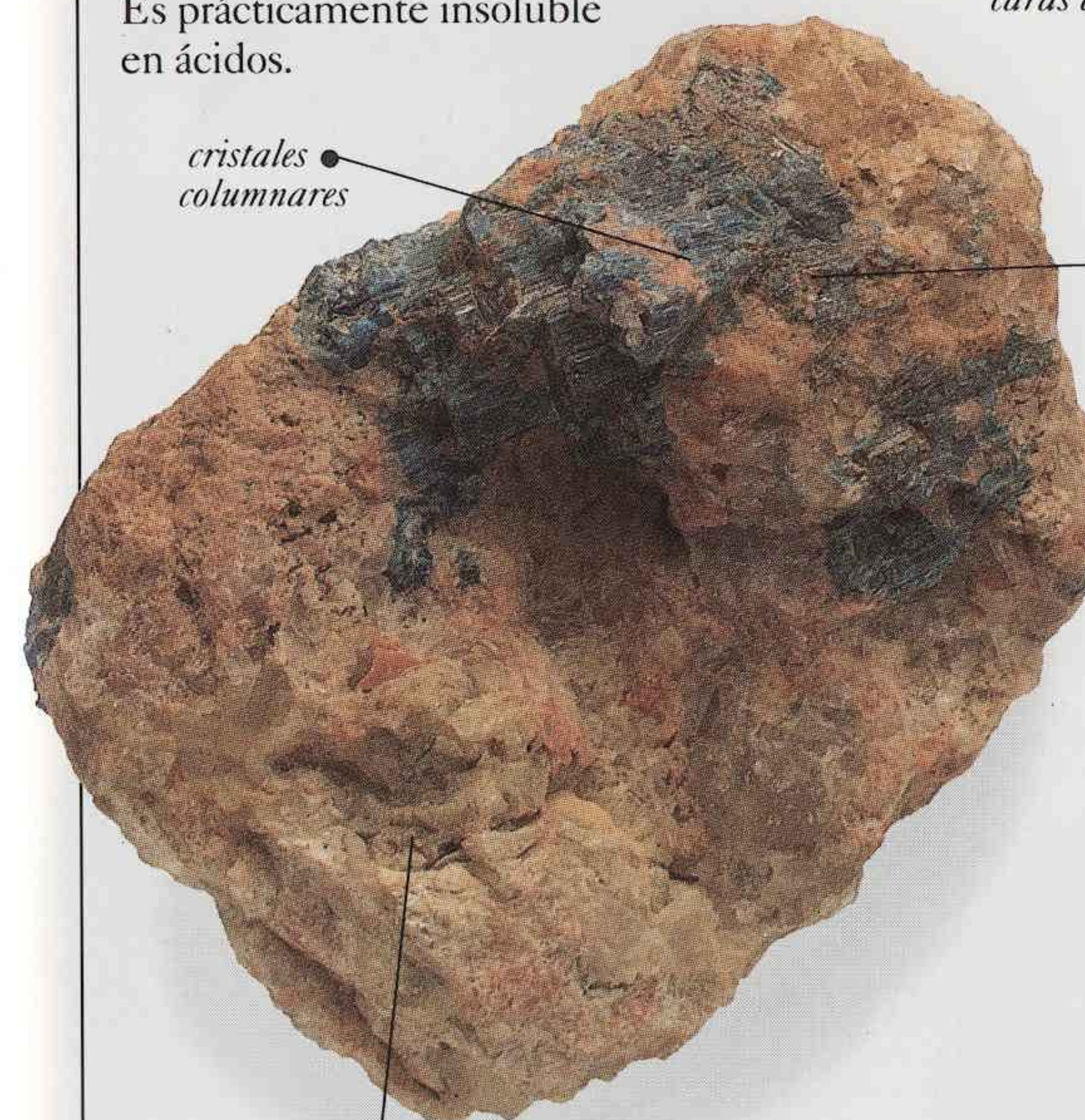
CIPRINA
