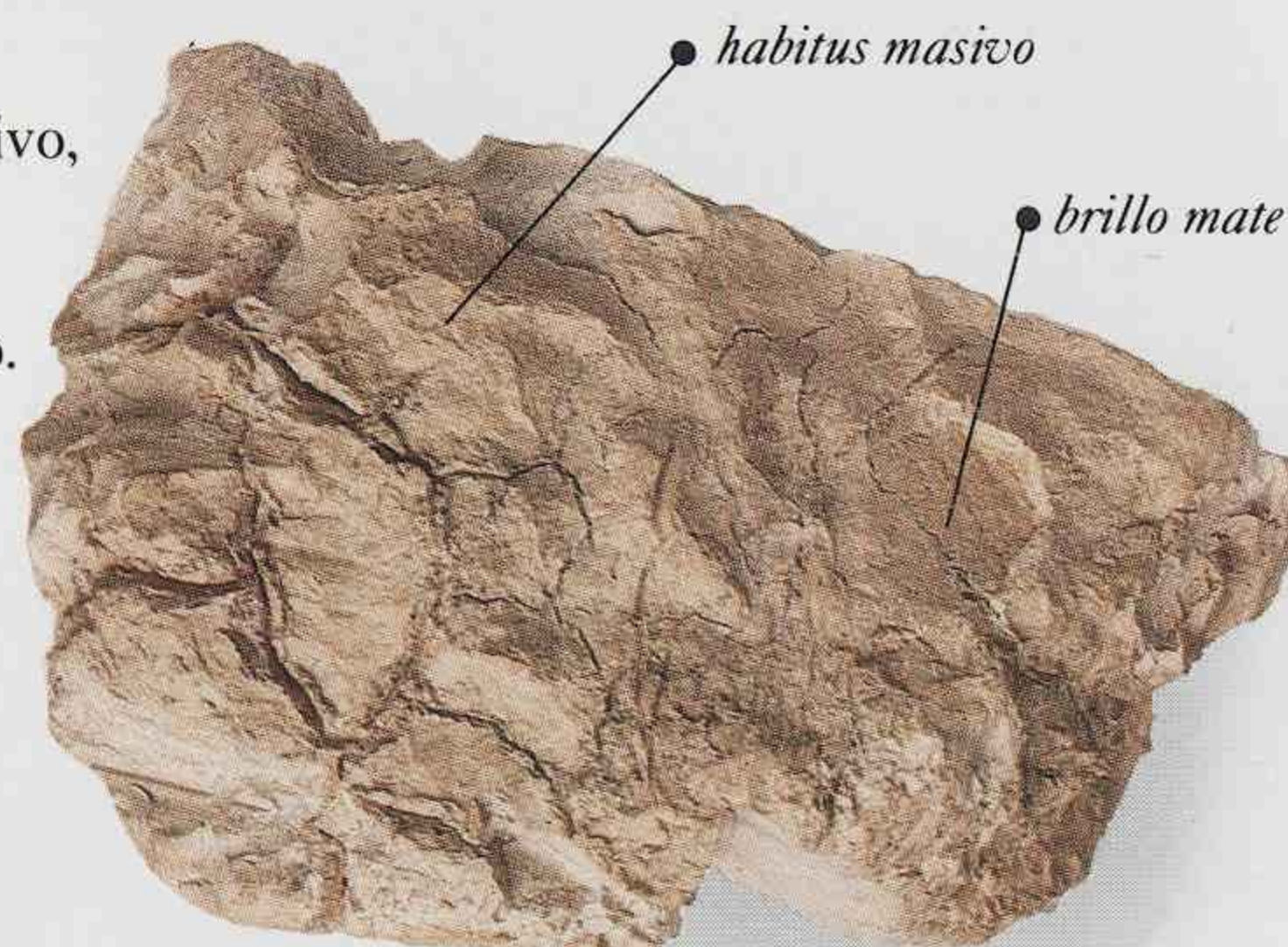
ROMBICO
