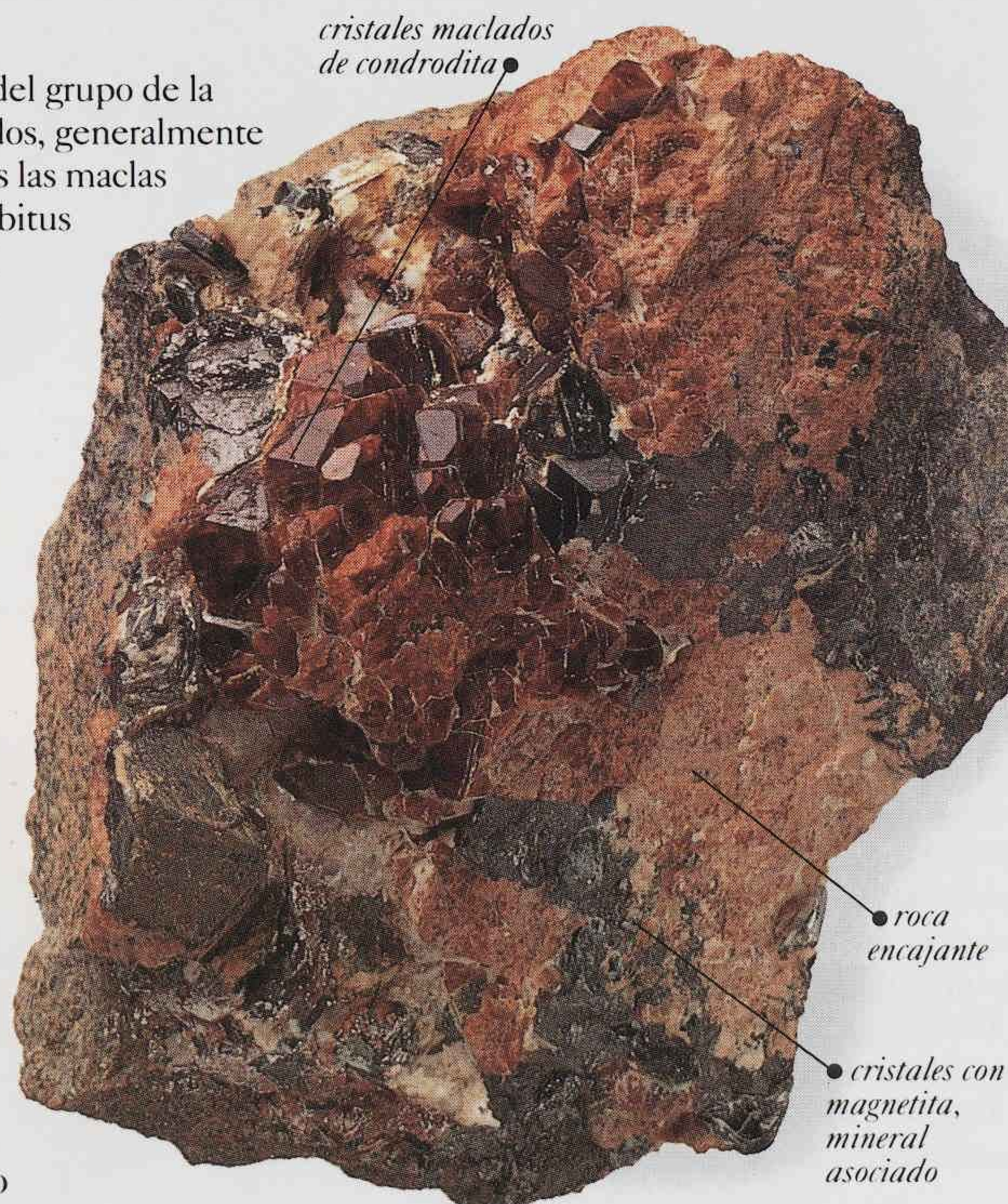
MONOCLINICO
