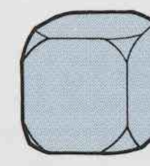
CUBICO
